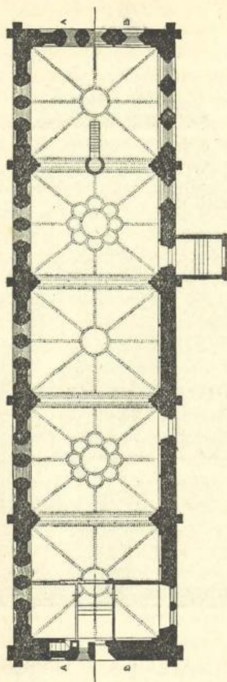
Platte grond der kerk.
