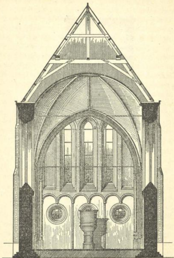
Dwarsdoorsnede der kerk, na haar restauratie, gezien naar het Oosten.
